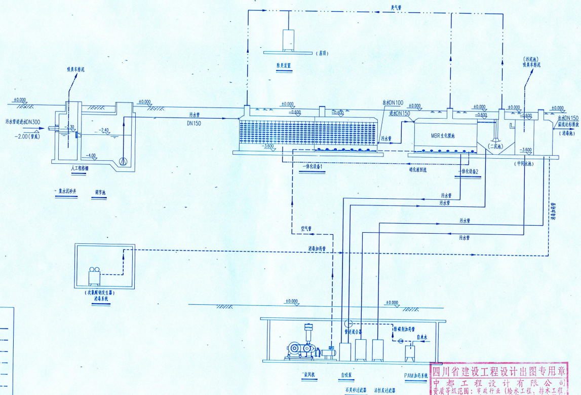
工艺流程图
